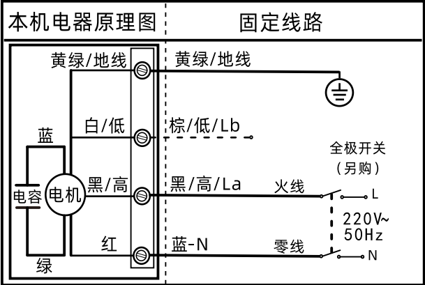
带双控开关电路图
