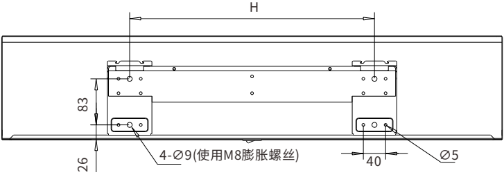
挂墙板尺寸图
