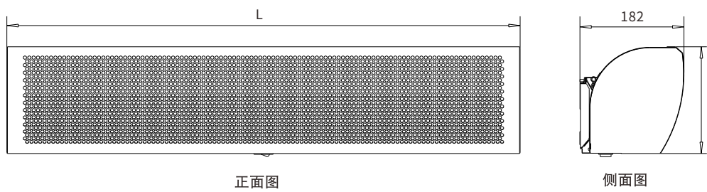
正面图
